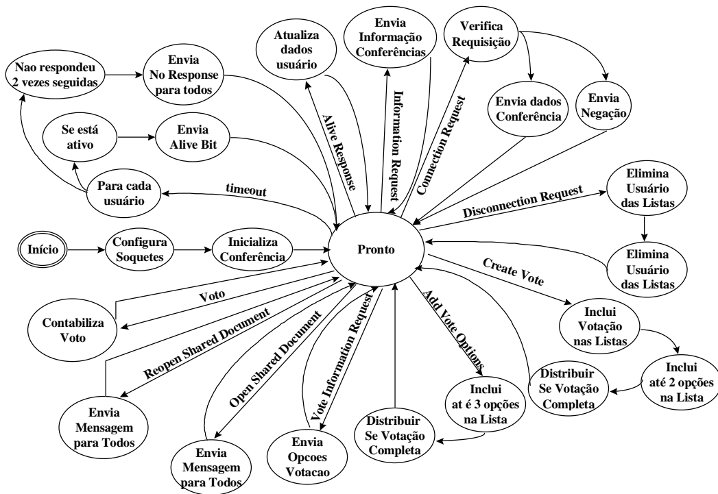
Figura 5.4: Diagrama de Estados do Daemon
