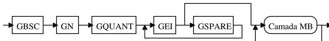
Figura 4.16: Camada GOB: Diagrama de Sintaxe
